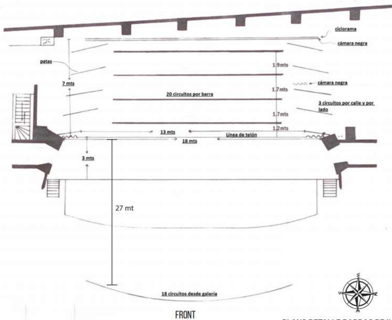
PLANO DETALLE BARRAS DE ILUMINACIÓN TEATRO POPULAR MELICO SALAZAR
